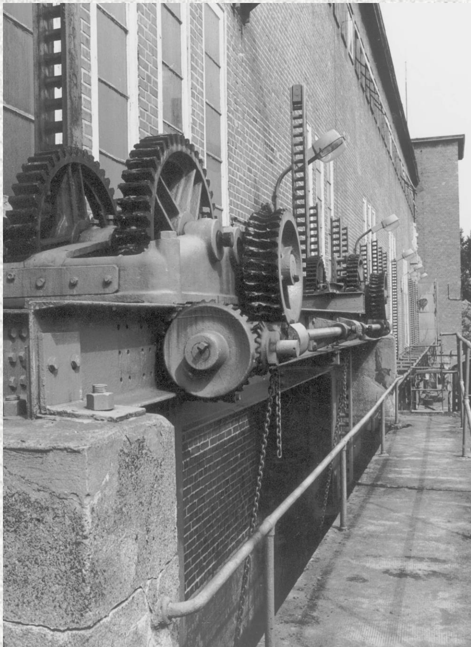
Elektrownia wodna Wrocław-Południe. Napędy zamknięć komór turbinowych 1922-1924
