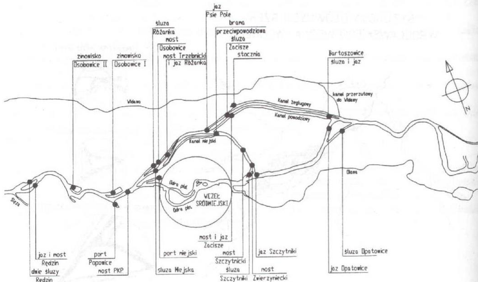
Układ przestrzenny wrocławskiego węzła wodnego, rys. R. Majewicz
