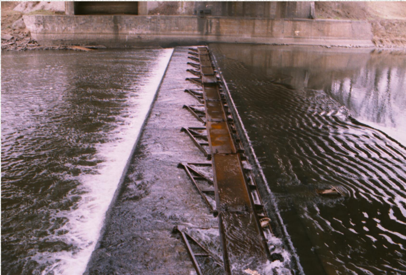
Jaz kozłowo-iglicowy Zacisze na Kanale Powodziowym we Wrocławiu.
